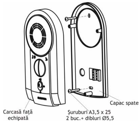
Fig. 5 Modul de amplasare a panoului exterior video
