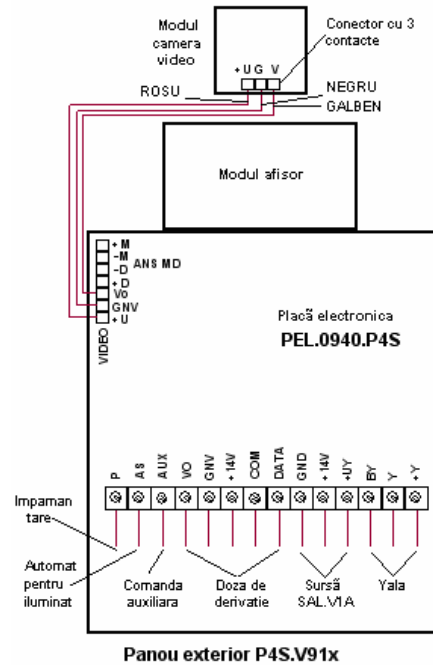
Fig. 27 Schema de conexiuni pentru upgrade panou exterior P4S.A91G
