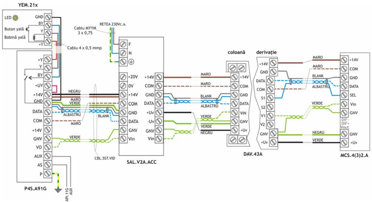
Fig. 12 Instalație ELECTRA PREMIUM - VIDEO, cu sursă de alimentare SAL.V2A.ACC și yală electromagnetă YEM.21x, realizată cu cablu CBL.5ST.VID
