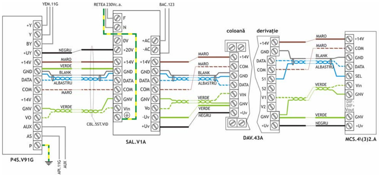
Fig. 11 Instalație ELECTRA PREMIUM - VIDEO, cu sursă de alimentare SAL.V1A și yală electromagnetă YEM.11x, realizată cu cablu CBL.5ST.VID
