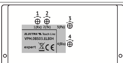
Vedere a modulului de comandă al panoului
