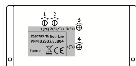
Vedere a modulului de comandă al panoului
